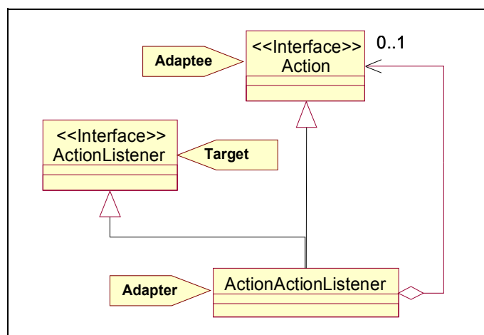
Abbildung 11 ActionActionListener kann sowohl als „class adapter“ als auch als „object adapter“ verwandt werden.
