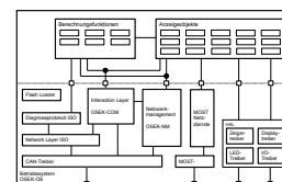
Software-Architektur
