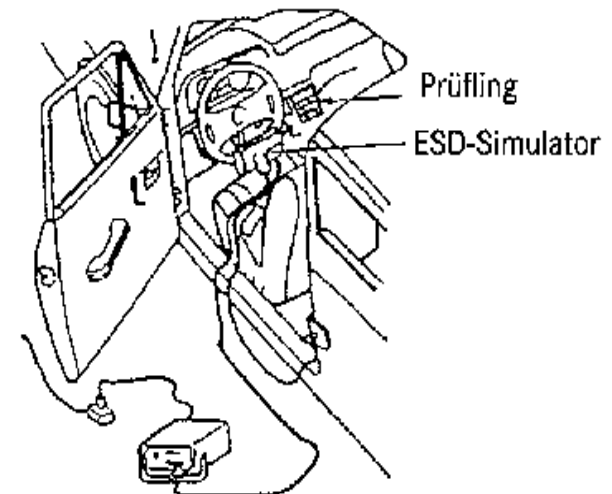
Prüfaufbau: ESD-Fahrzeugprüfung nach ISO/TR 10605
